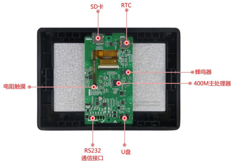
图 1-2 硬件配置图
