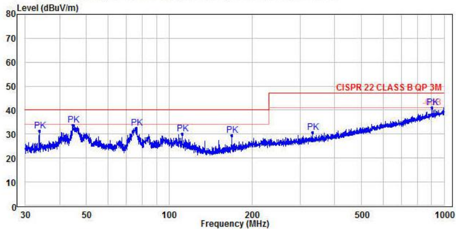
图 5-6 RE 测试垂直方
