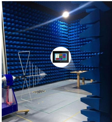
图 5-4 RE 测试图
